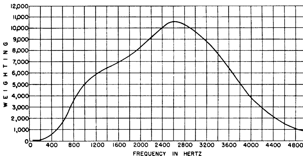
Figure 6-2—1960 TIF Weighting Values
